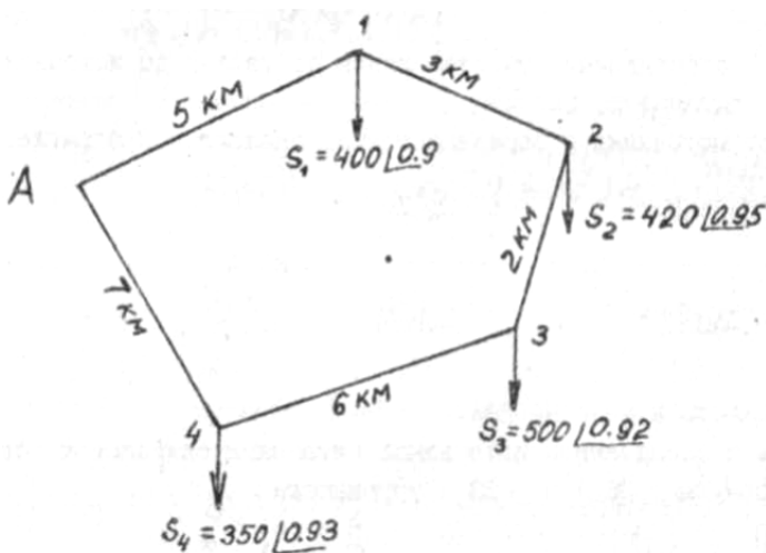
Рис 1. Схема сети 10 кВ.
