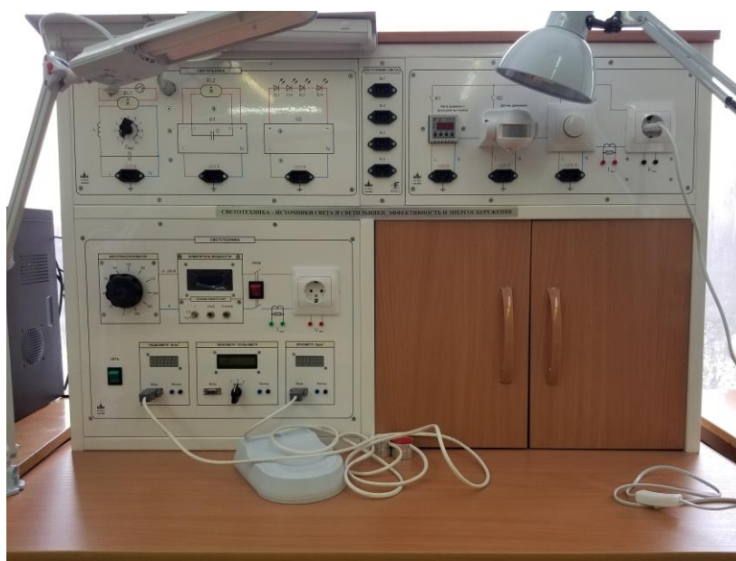
Рисунок 2 – Стенд для занятий по строительной физике
