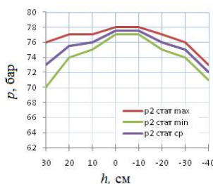
Рис. 1.2. Распределение статического давления
