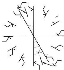
Рис.9 Примеры нанесения условных обозначений шероховатости
