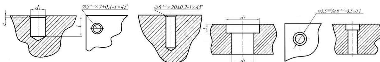
Рис.21 Обозначение размеров отверстий
