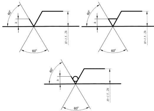
Рис.8 Знаки обозначения шероховатости поверхности
