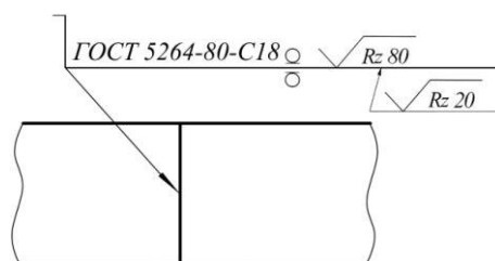
Рис.13 Условное обозначение сварного шва
