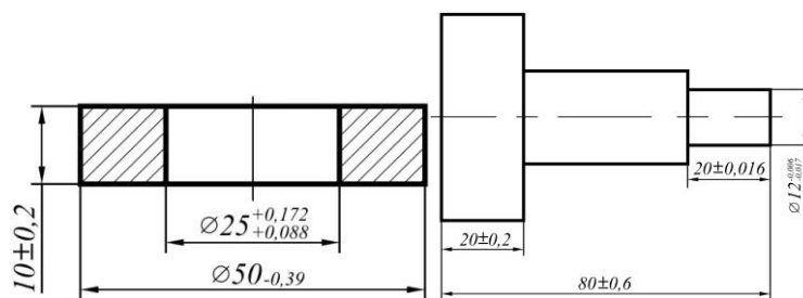
Рис.18 Обозначение предельных отклонений линейных размеров
