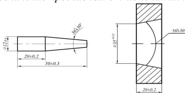
Рис.19 Обозначение угловых размеров с отклонениями
