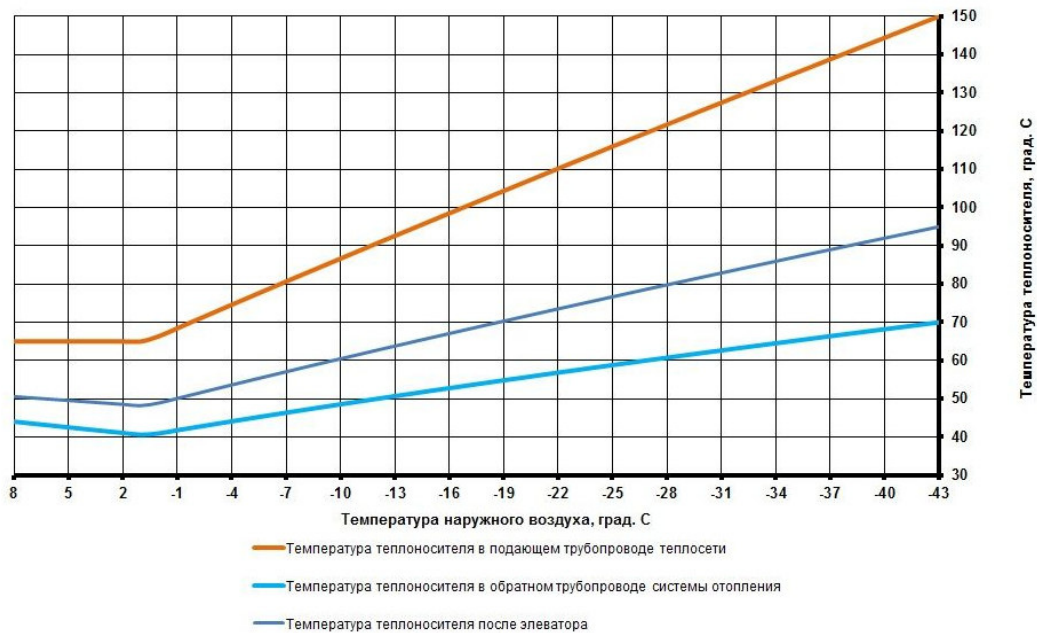
Рис. 3.1 Температурный график 150-70 0 С со срезкой на ГВС
