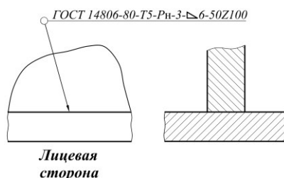
Рис.14 Условные обозначения некоторых видов сварных швов
