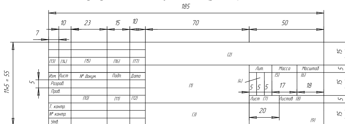
Рис.1 Форма 1 основной надписи для чертежей и схем
