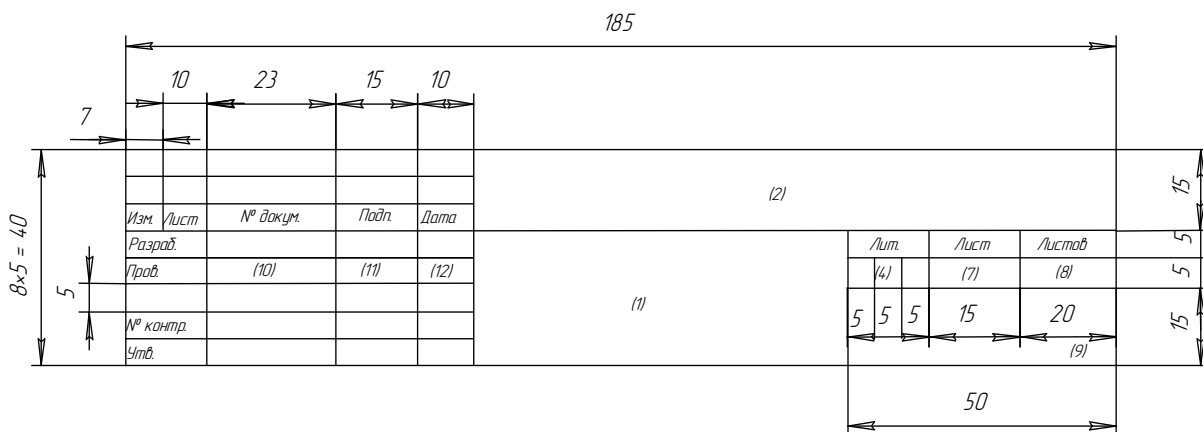
Рис.2 Форма 2 основной надписи для текстовых документов (графиков, диаграмм, таблиц и т.п.)
