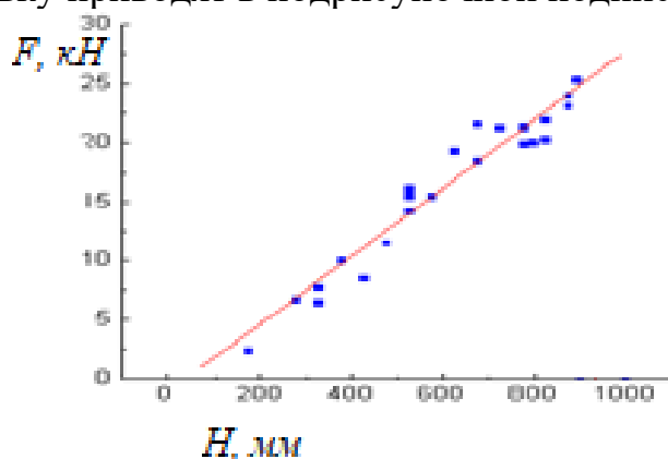
Рис. 3.1 Зависимость тягового усилия от глубины копания
