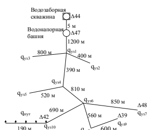
Схема систем водоснабжения
