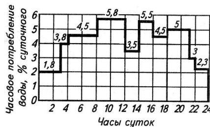
График суточного водопотребления
