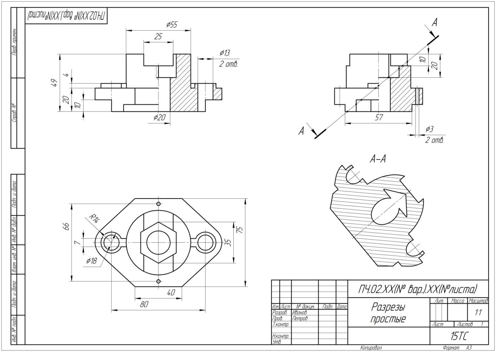
Рис.4. Простые разрезы.
