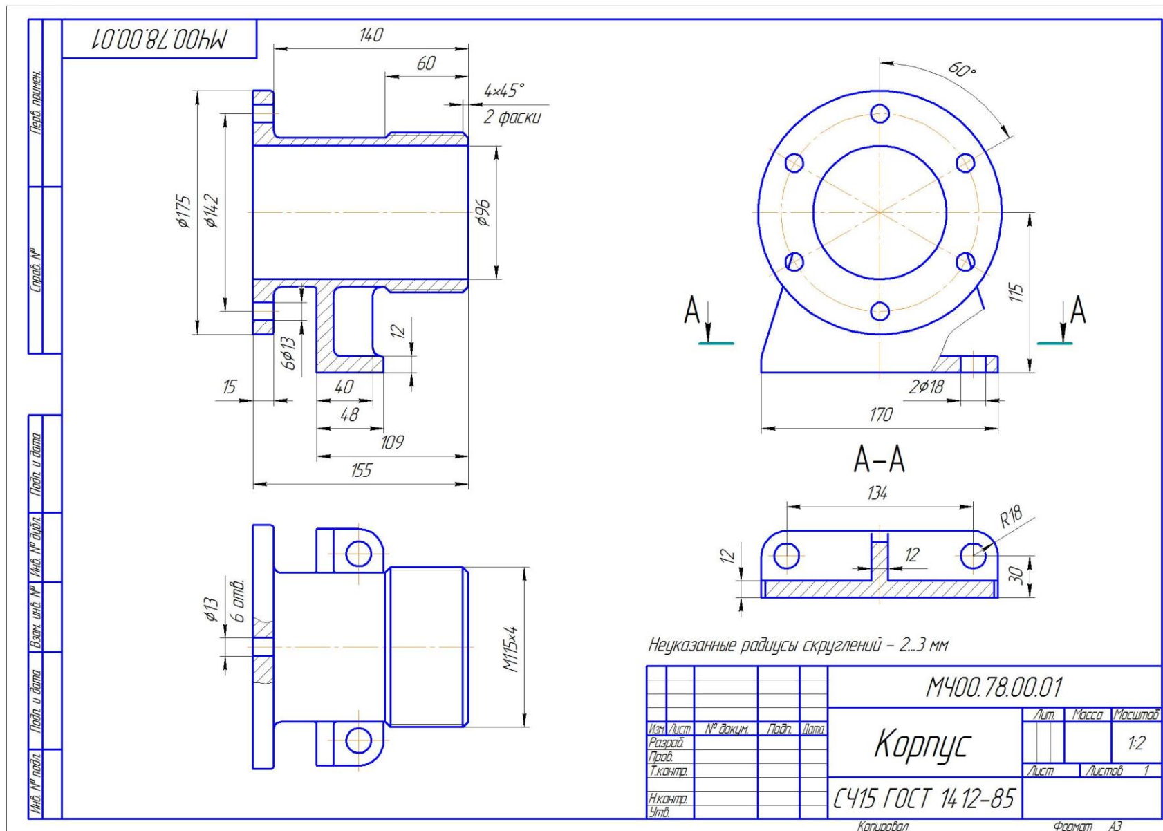
Рис. 10. «Деталирование». Чертежи деталей.
