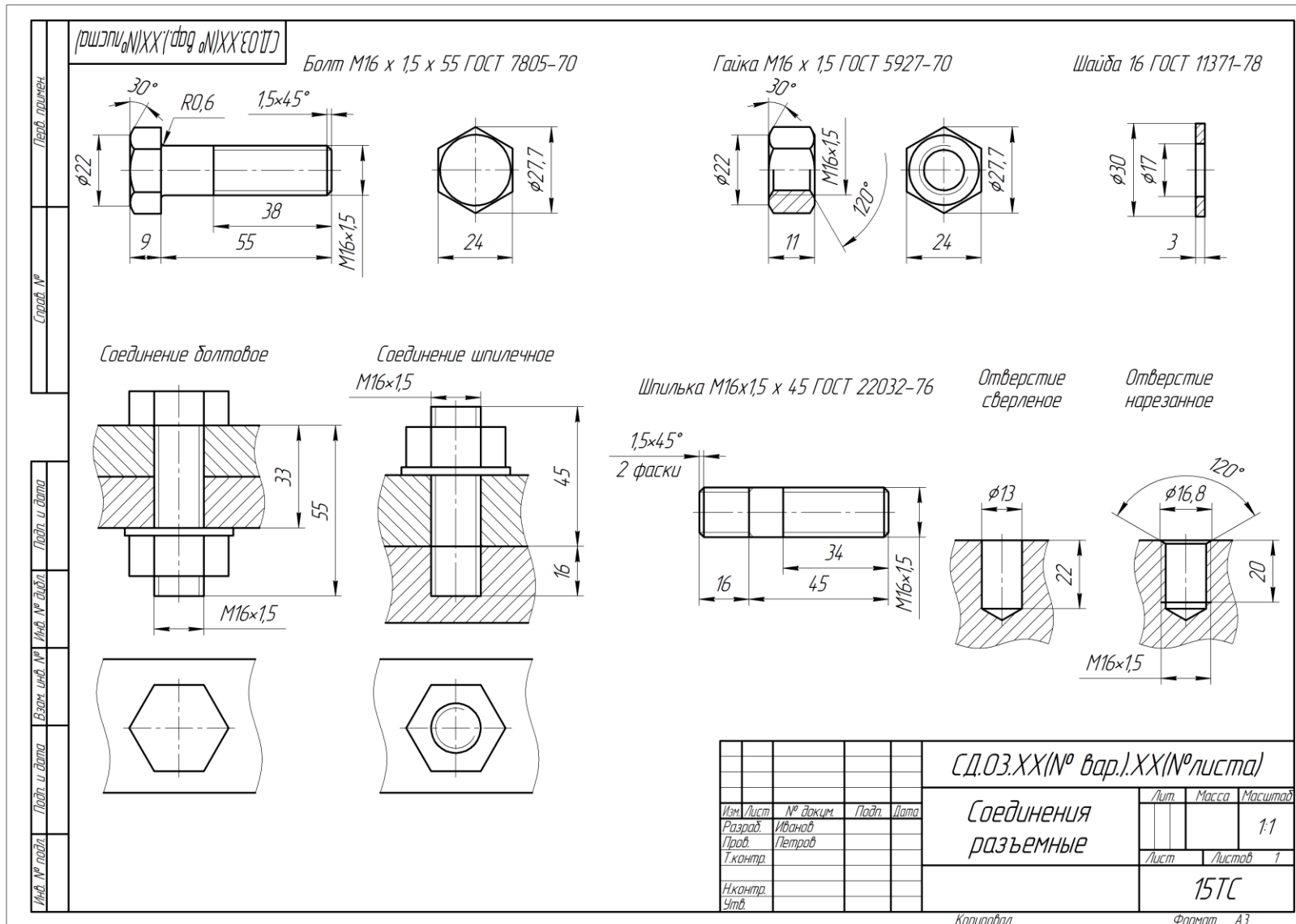
Рис. 7. Соединения разъемные резьбовые.
