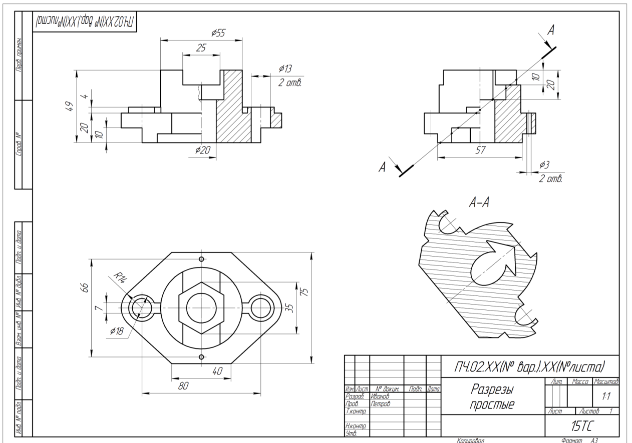
Рис. 4. Простые разрезы.
