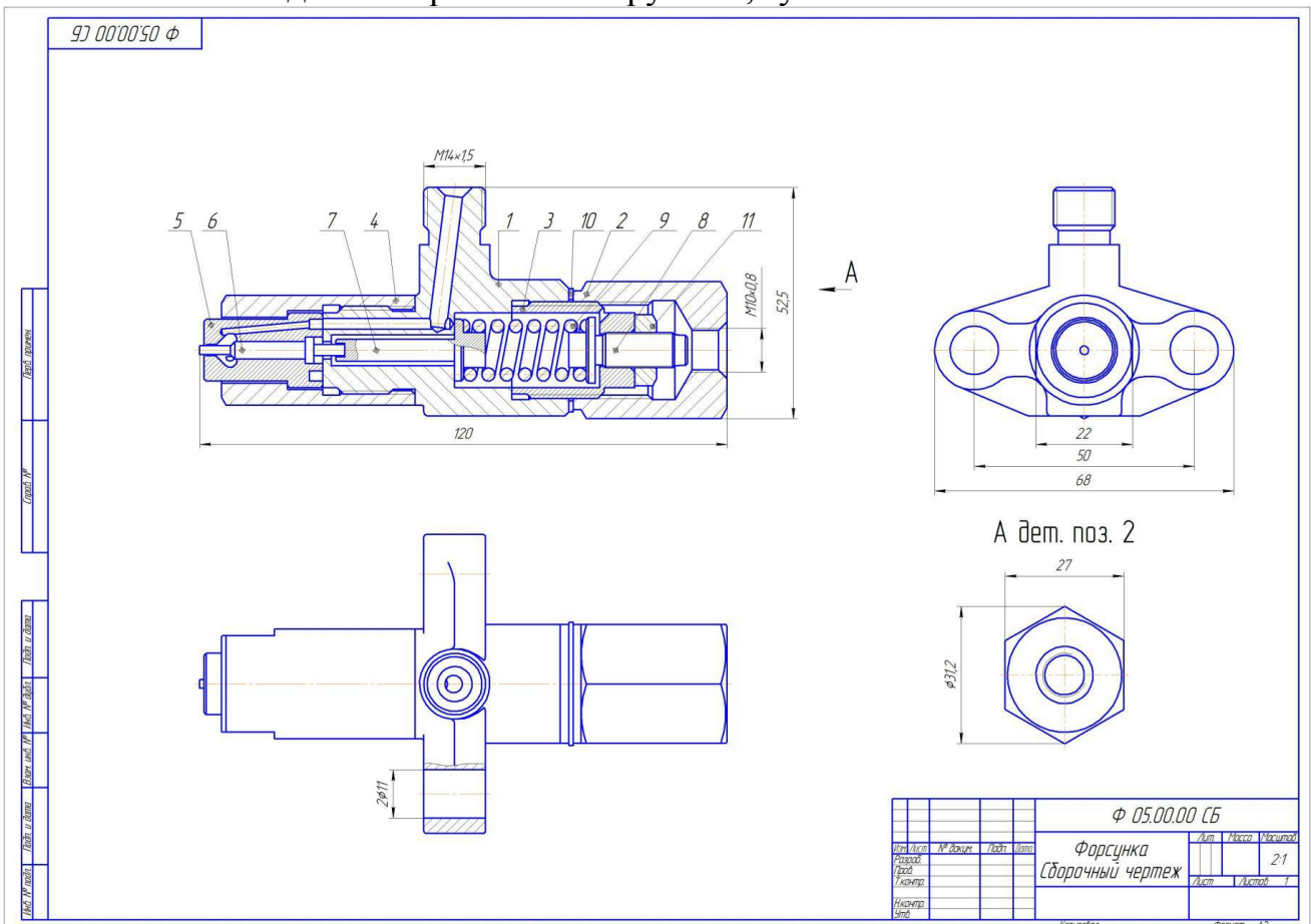
Рис. 10. Чертеж общего вида.
