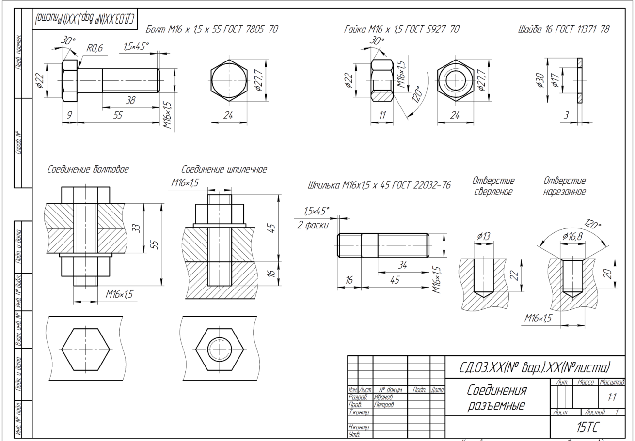
Рис. 8. Соединения резьбовые разъемные.
