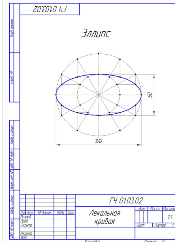
Рис. 1. Сопряжения. Лекальная кривая.
