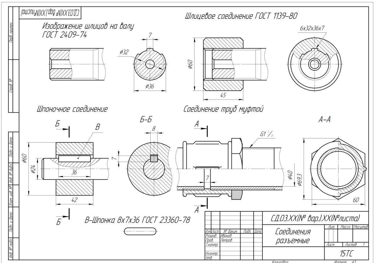
Рис. 9. Соединения разъемные трубные, зубчатые и шпоночные.
