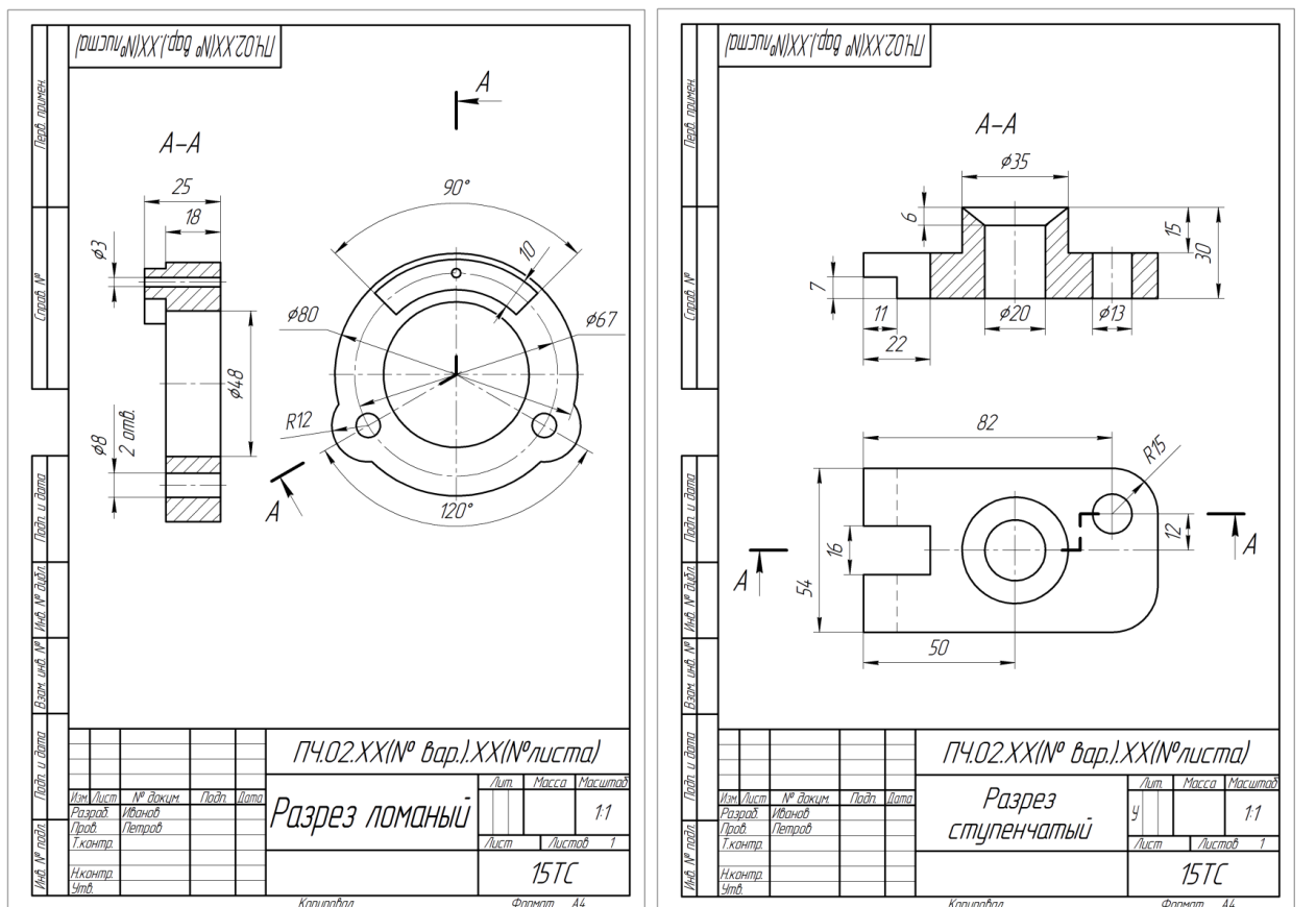
Рис. 5. Сложные разрезы.
