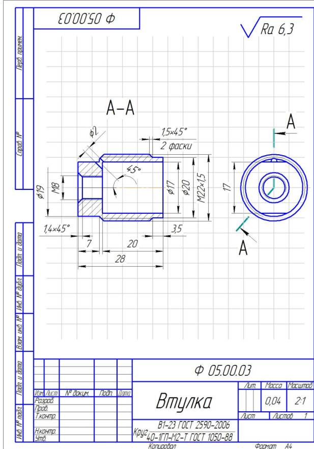
Рис. 11. Спецификация. Эскизы.
