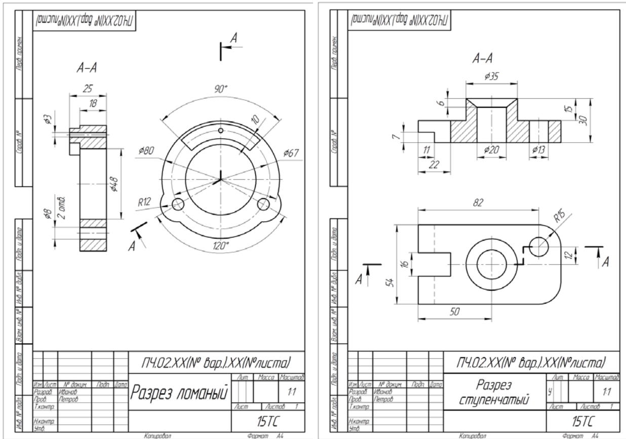
Рис. 9. Сложные разрезы.
