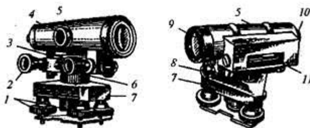
Рисунок 7. Нивелир Н-3.
