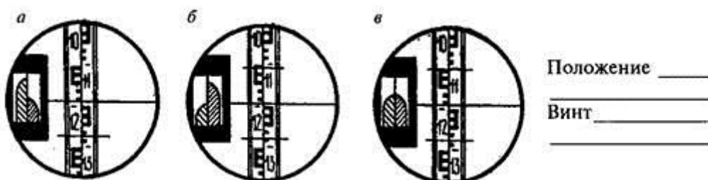
Рис. 8. Изображение пузырька цилиндрического упроня в поле зрения трубы нивелира Н-3.
