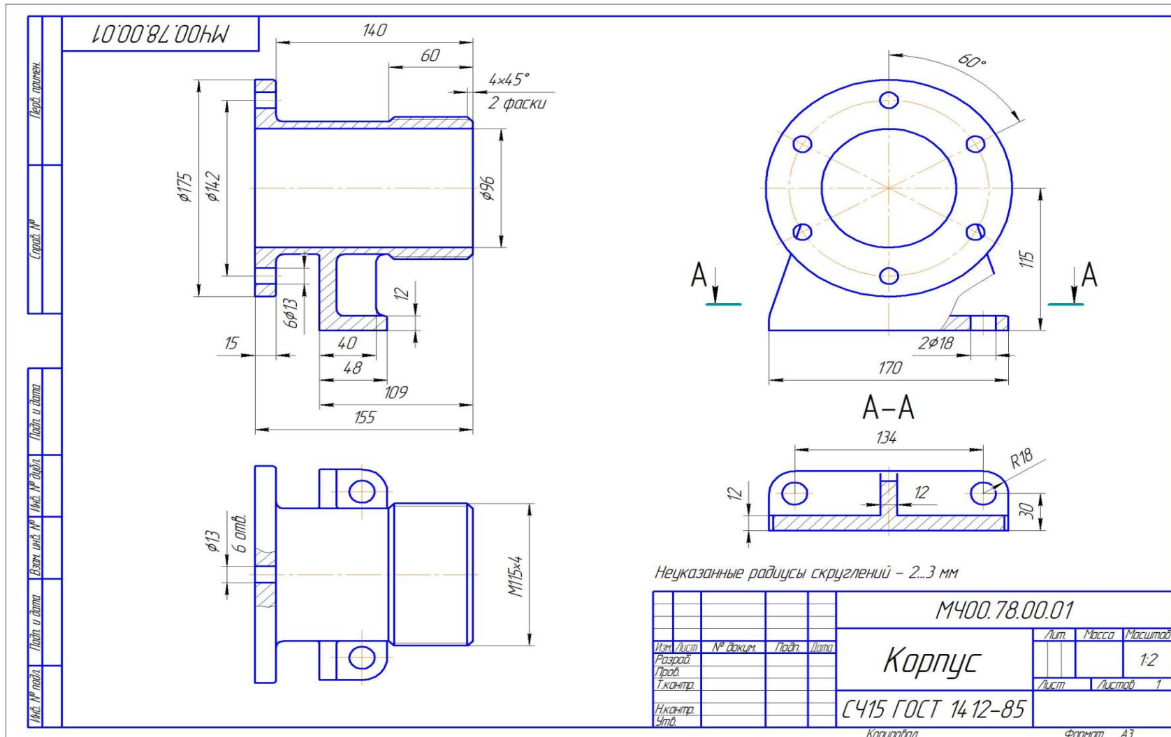
Рис. 13.Образец выполнения графической работы №2 «Деталирование». Чертежи деталей.
