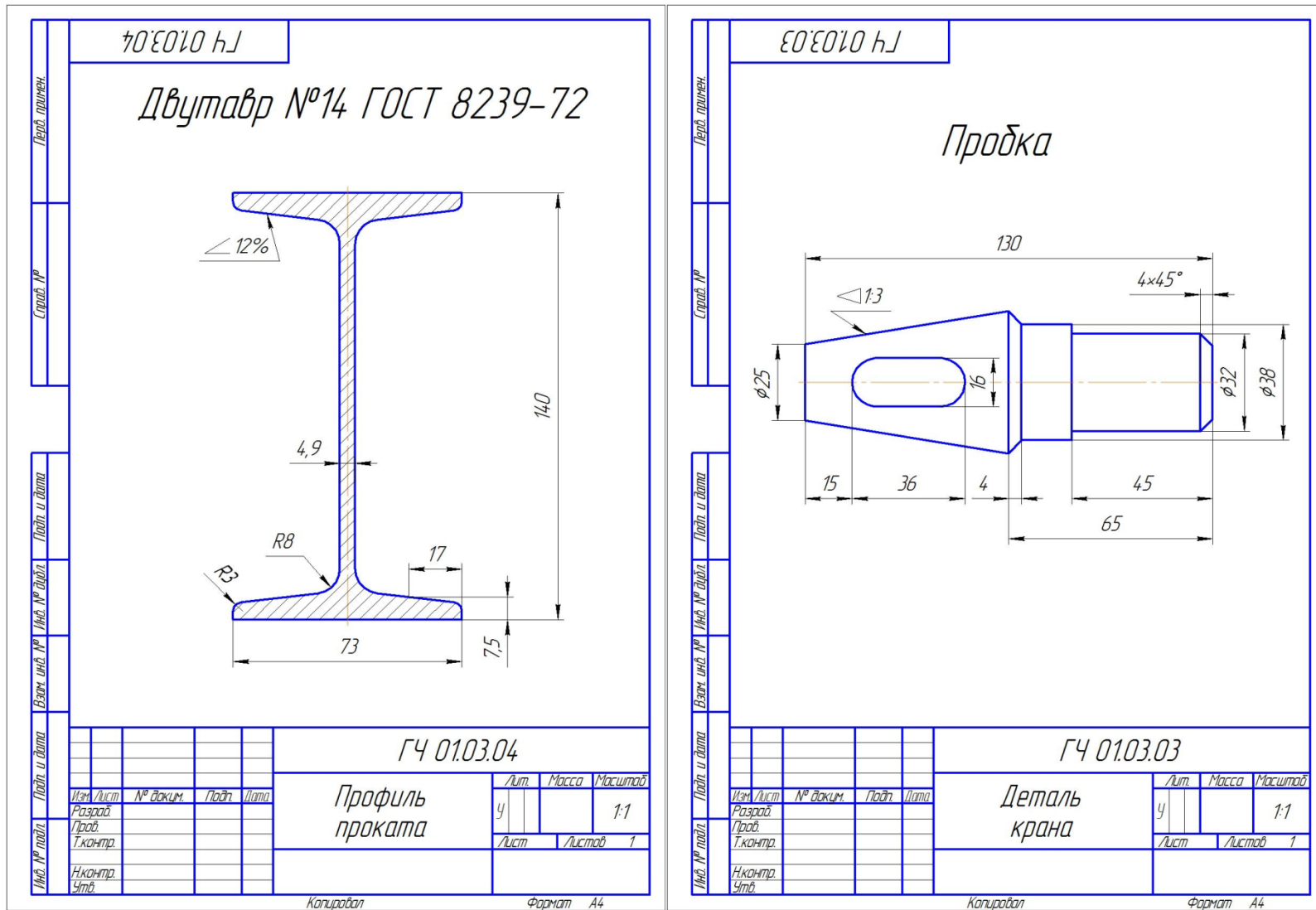
Рис12.Образец выполнения графической работы №1 по теме Конусность. Уклон.
