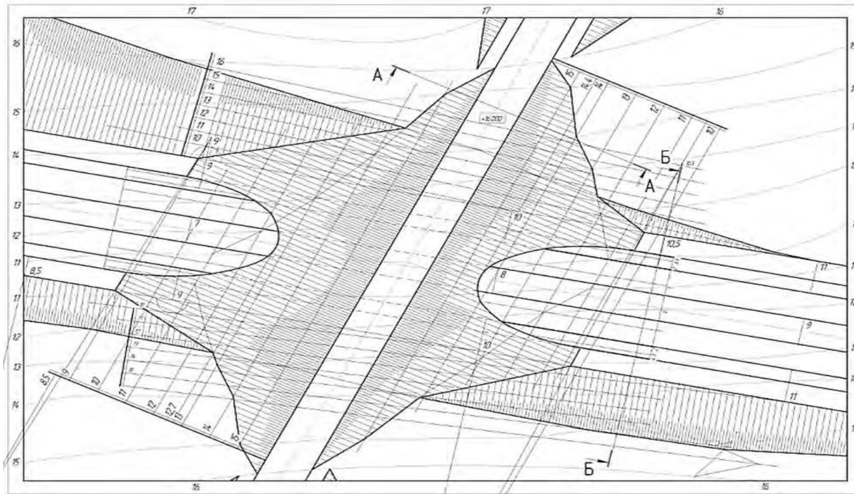
Рис. 15. Образец выполнения графической работы №4 «Привязка сооружения к топографической поверхности»
