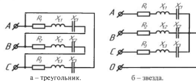
Рис. 2. Трехфазная цепь соединении потребителей звездой или треугольником.
