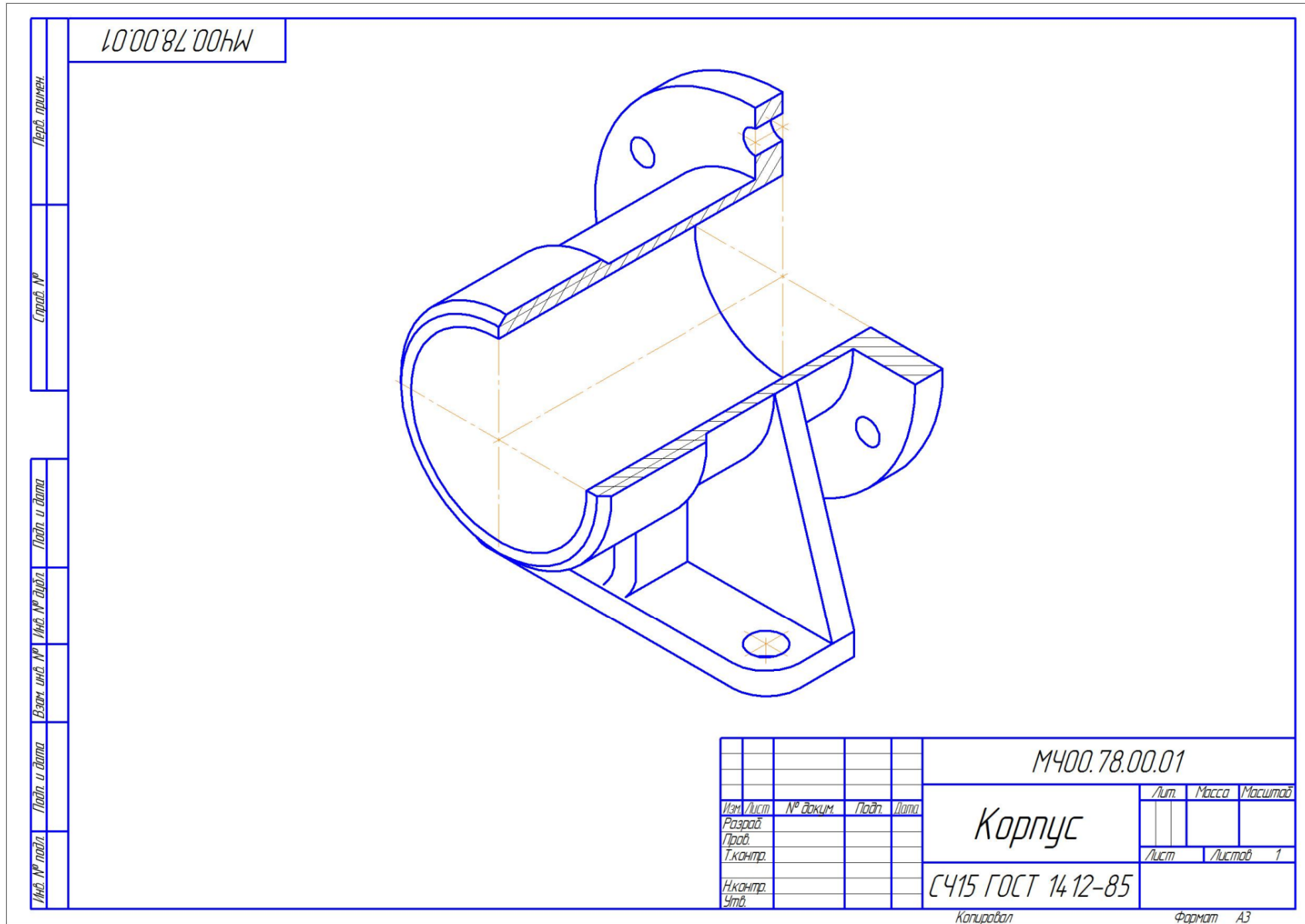
Рис. 10. Графическая работа «Детализация чертежа» (Лист 12 – Изометрия корпусной детали)
