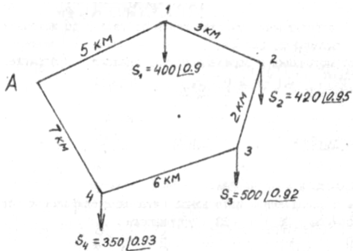
Рис 1. Схема сети 10 кВ.
