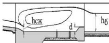
Водобойная стенка
