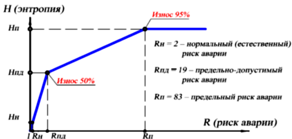
Рис. 1 Модель деградации несущего каркаса объекта и пороговые значения риска аварии
