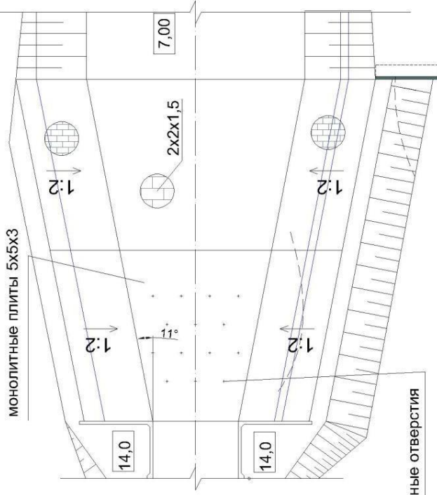
Конструкция рисбермы 1:500
