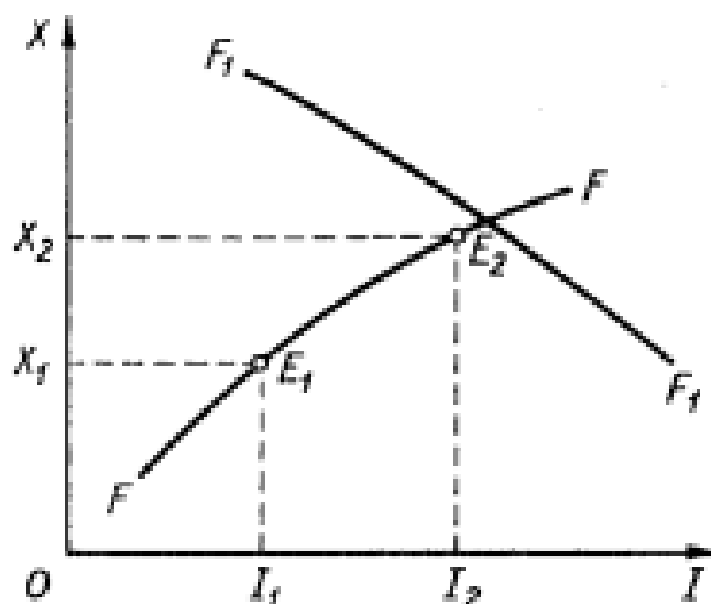
Рисунок 3.1 - Кривая Энгеля
