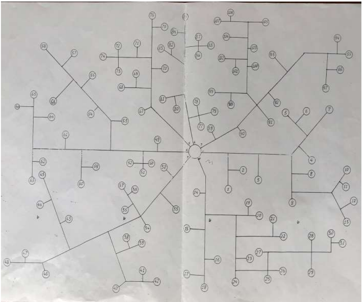
Рисунок 1—Схема фидеров 10 кВ, отходящих от РТП 110/10 кВ
