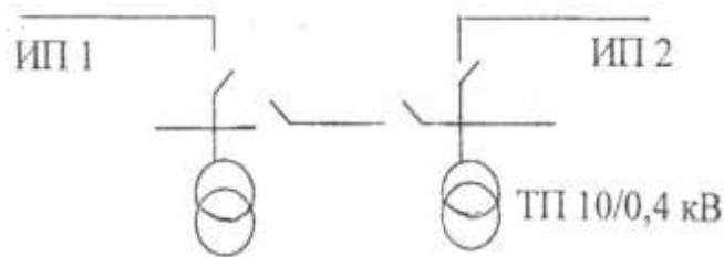
Рисунок 11 – Схема присоединения ТП 10/0,4 кВ, питающей потребителей второй категории с расчетной нагрузкой 120 кВт и более
