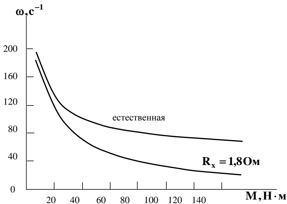
Рисунок 2 – Механические характеристики электродвигателя
