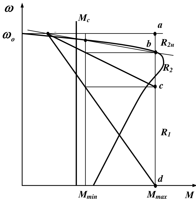
Рисунок 2 – Пусковая диаграмма
