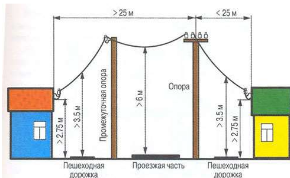
Рисунок 1 – Нормативные размеры
