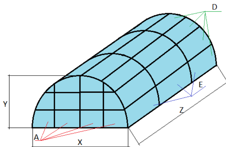
Рисунок 1 – Вид сбоку и спереди теплицы из поликарбоната
