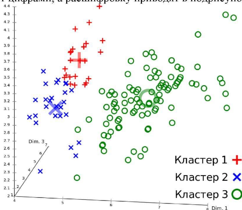
Рис. 3.1 Метод k -средних
