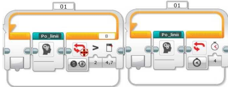
Рис. 8. Цикл с энкодером мотора (слева) и по времени (справа)
