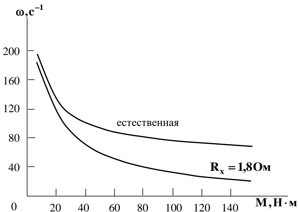
Рис. 3.1. Естественная и реостатная механические характеристики двигателя
