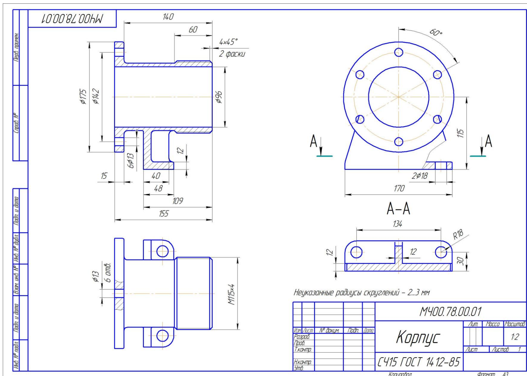
Рис. 9. Графическая работа «Детализирование чертежа» (Лист 11 – Чертежи деталей)
