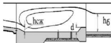
Водобойная стенка
