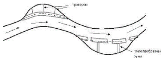
Выправление русла с помощью продольных сооружений
