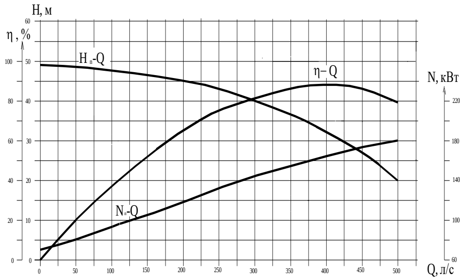
Характеристика насоса Д –1000 - 40 (14НДс), n = 980 об/мин
