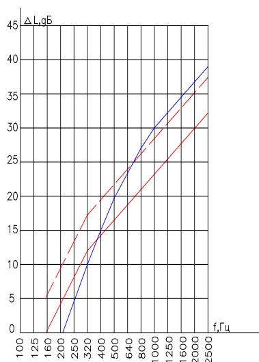
Рис. 3.1 Частотная характеристика требуемого снижения приведенного уровня ударного шума
