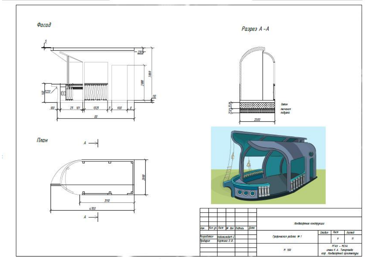
Рисунок 4. Проект парковой беседки
