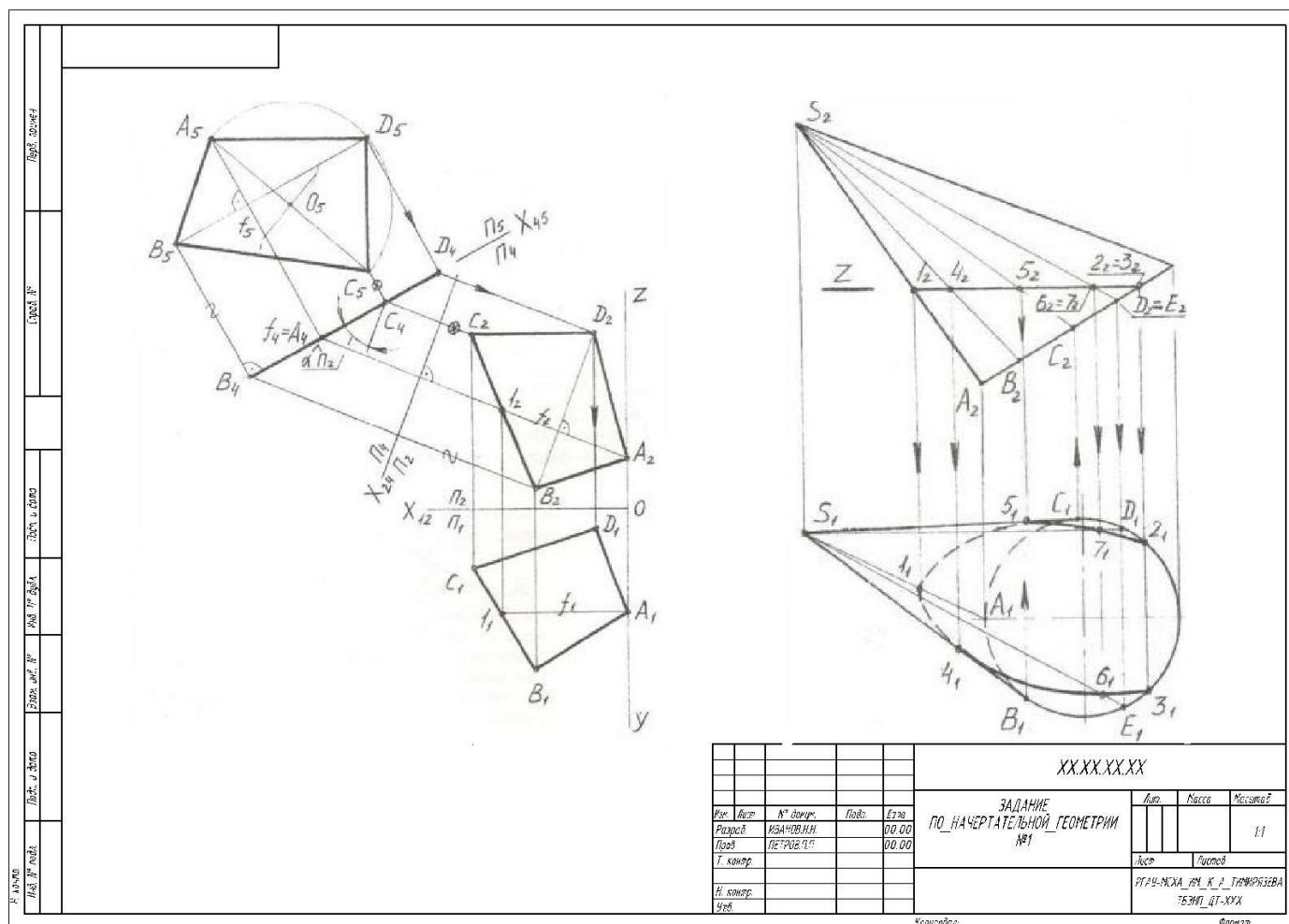
Рис. 3. Образец выполнения графической работы №1 по теме «Инцидентность точки, линии, поверхности»
