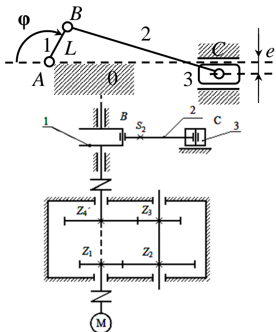
Структурные схемы привода и исполнительного механизма
