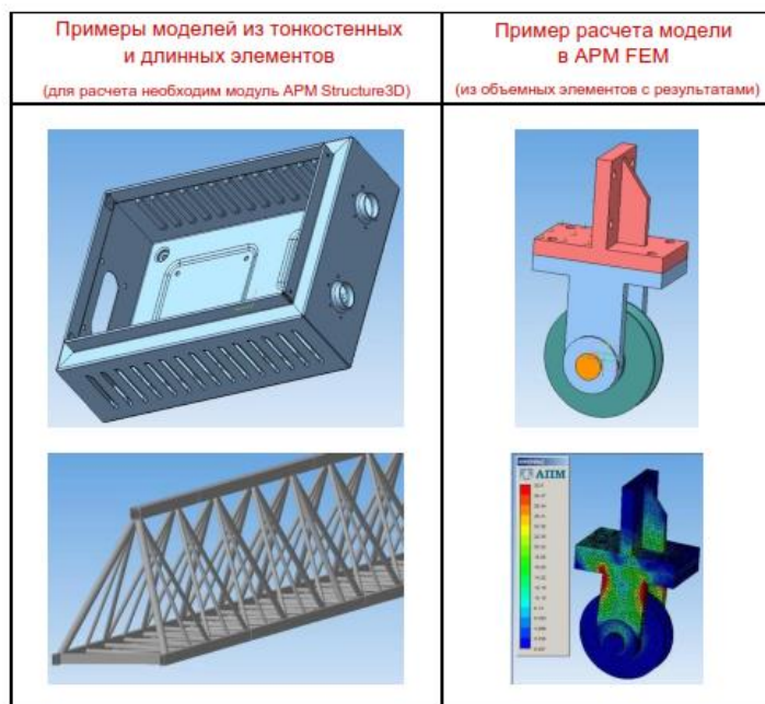
Рис. 5. Прочностной анализ
