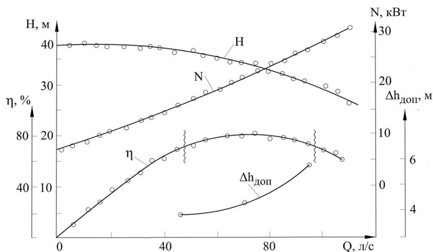
Рис. 3.1 Характеристики насоса, построенные по результатам испытаний
