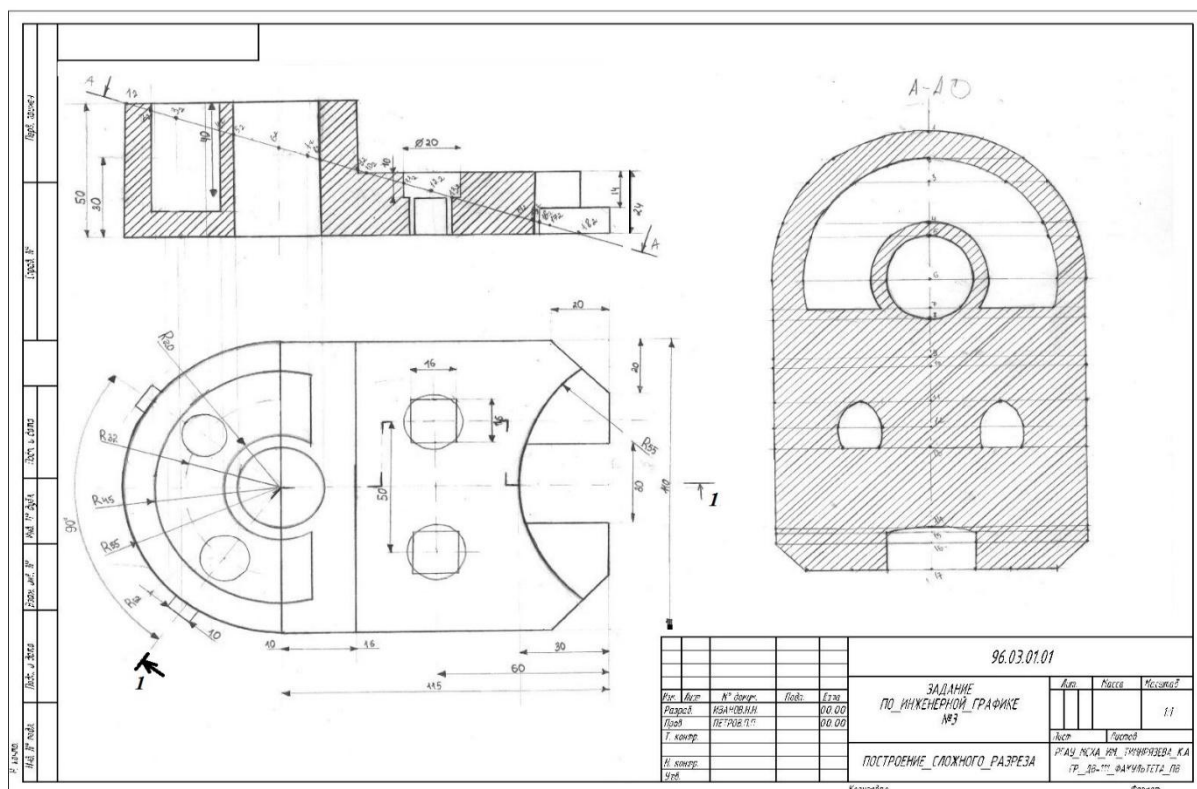
Рис. 10. Образец выполнения графической работы №2. Построение сложного разреза.
