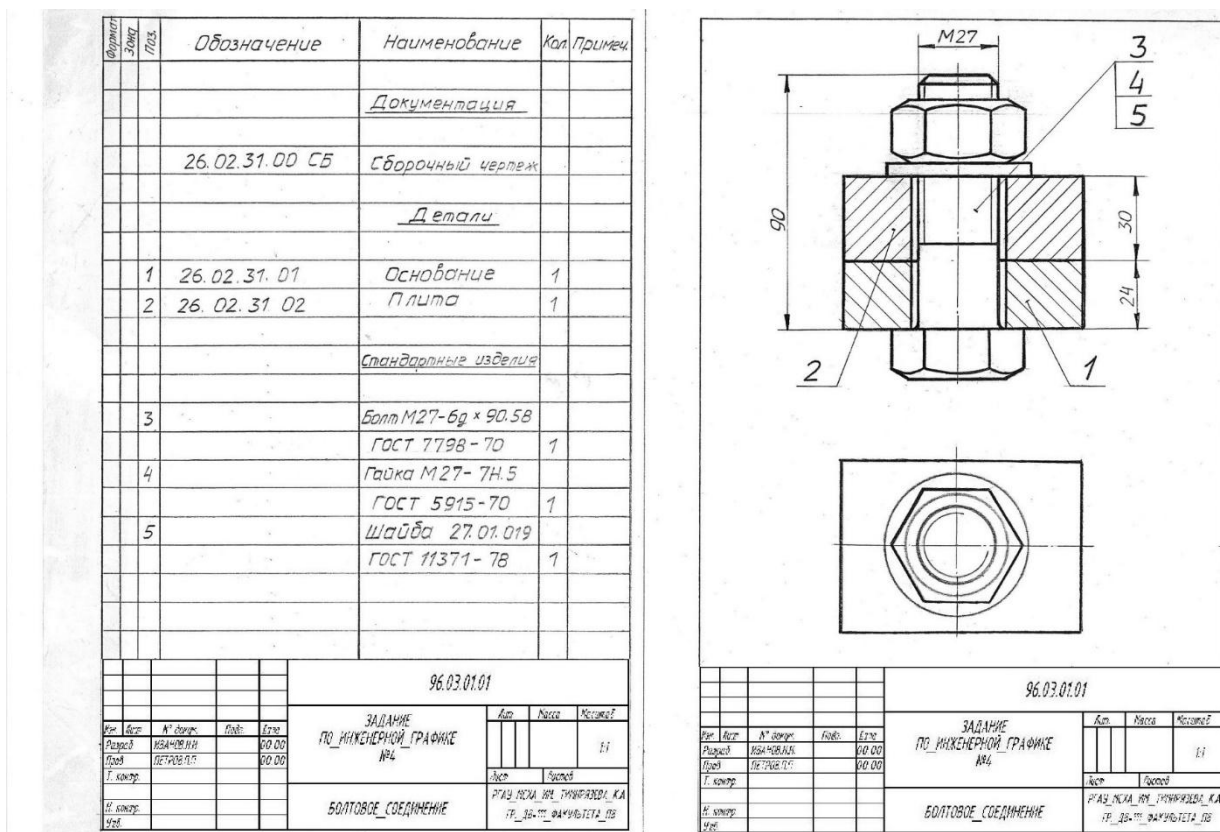
Рис. 11. Образец выполнения графической работы №3 по теме «Соединение деталей»
