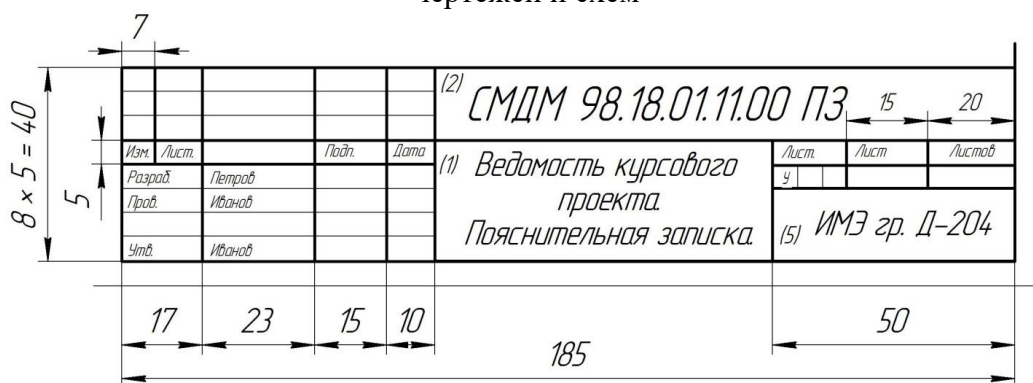
Рис. 5. Основная надпись по ГОСТ 2.104-68 для первого листа текстовых документов и
