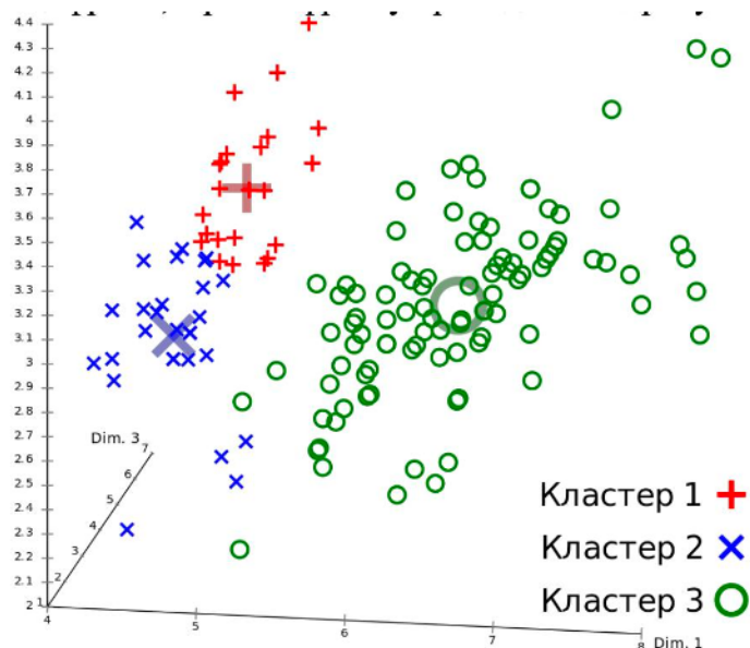
Рис. 3.1 – Метод k-средних
