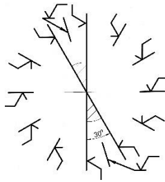
Рис.9 Примеры нанесения условных обозначений шероховатости
