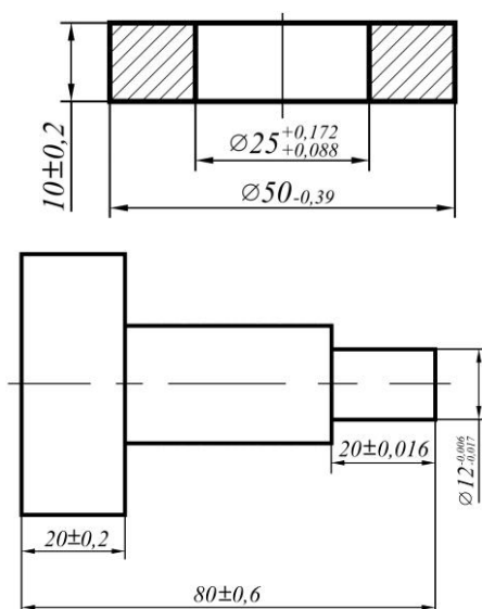
Рис.18 Обозначение предельных отклонений линейных размеров
