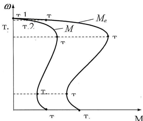
Рисунок 3 – Естественная и искусственная механические характеристики
