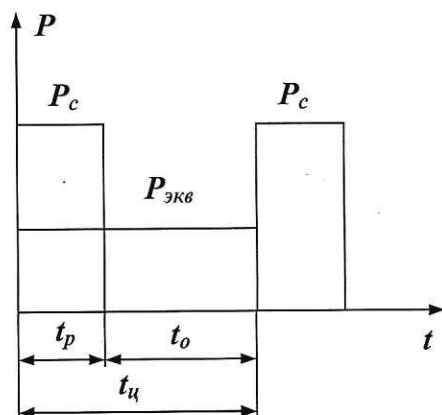
Рисунок 1 – Нагрузочная диаграмма
