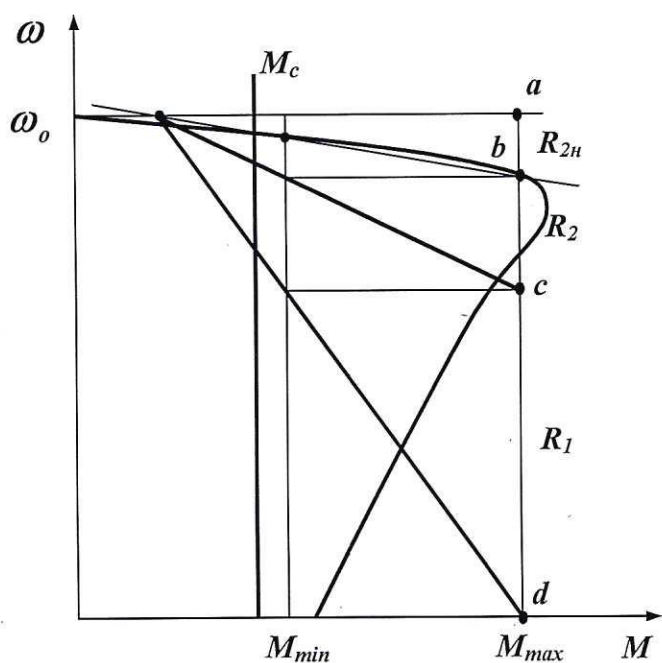
Рисунок 2 – Пусковая диаграмма
