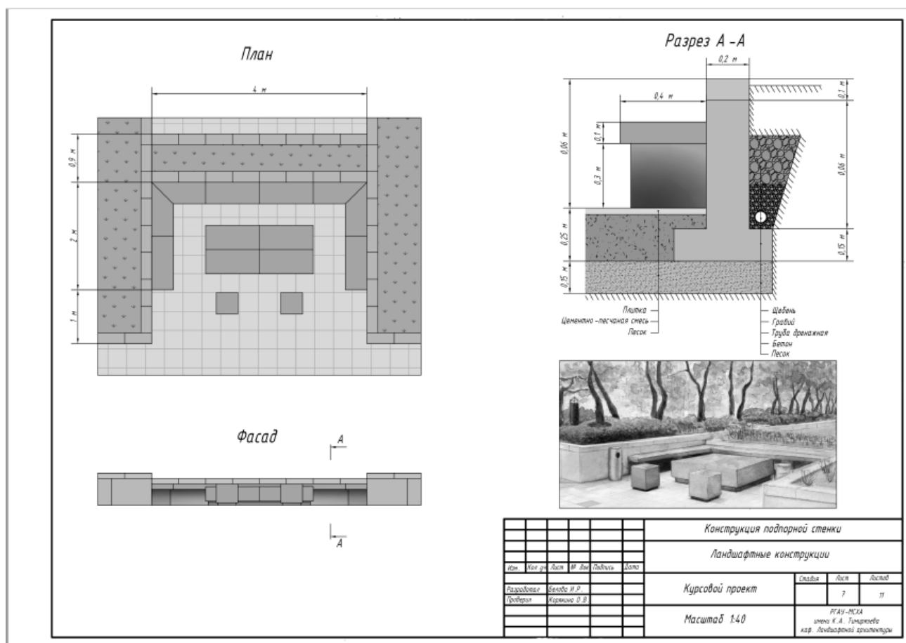
Рисунок 2 . Проект подпорной стенки
