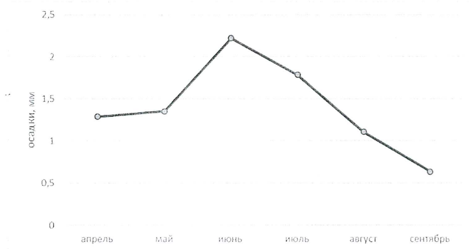
Рисунок 3.1 - Среднее количество выпавших осадков
