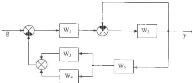
Рис. 1. Структурная схема САУ
