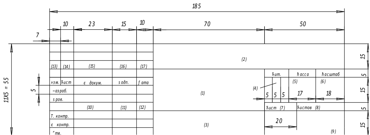
Рисунок 2.5 – Форма 1 основной надписи для чертежей и схем по ГОСТ 2.104-2006
