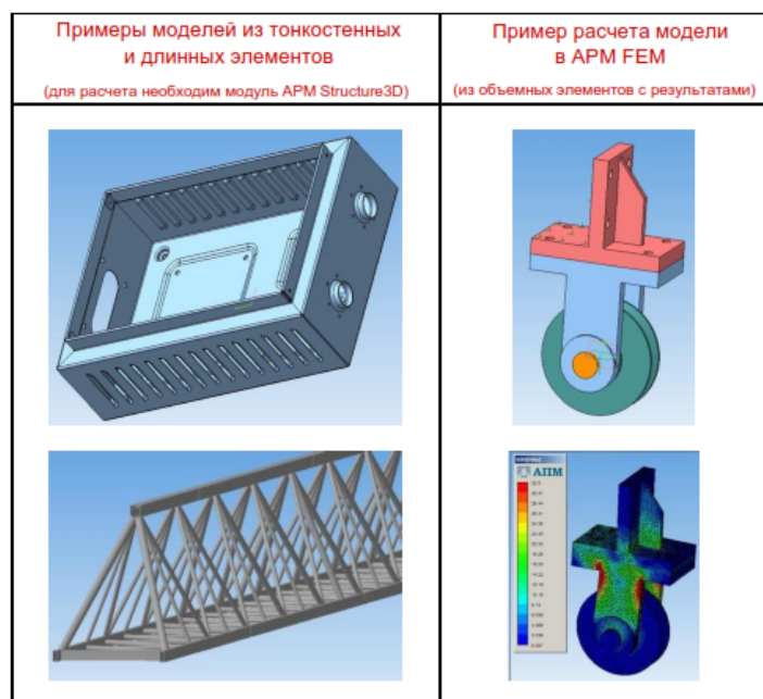
Рис. 5. Прочностной анализ
