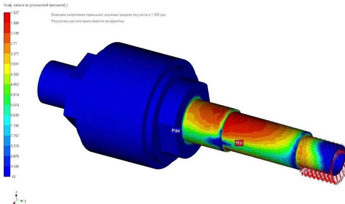
Рис. 4. Пример выполнения задания по разделу «Прочностной анализ в APM FEM»
