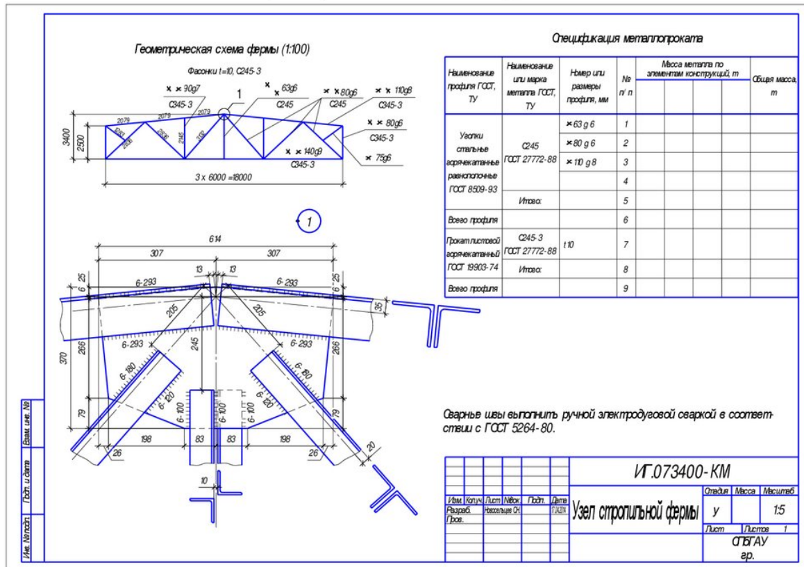
Рис. 2. Пример выполнения задания по разделу «Металлоконструкции»
