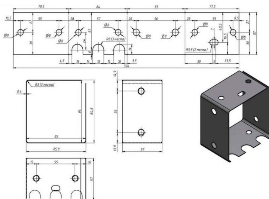
Рис. 1. Пример выполнения задания по разделу «Листовое моделирование»
