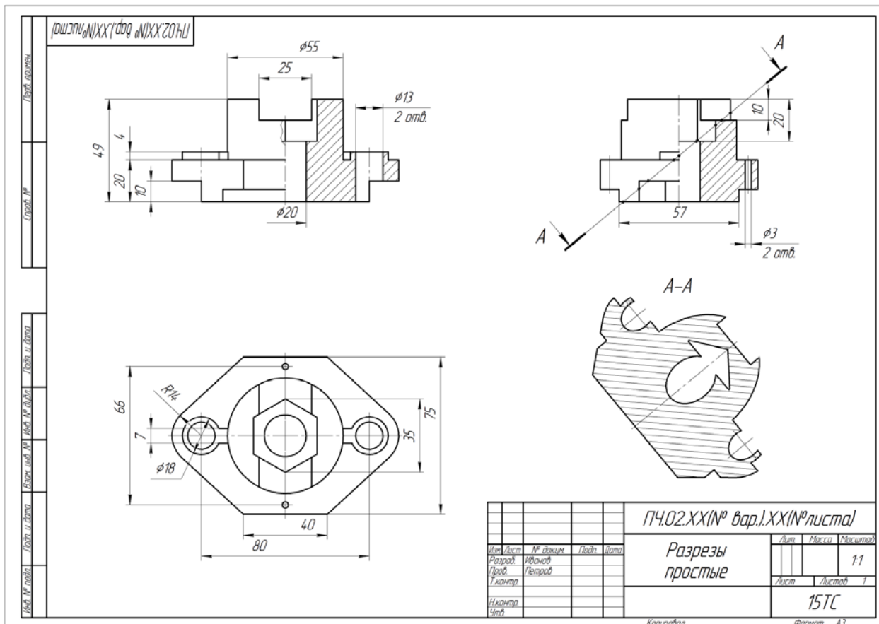
Рис. 4. Простые разрезы.
