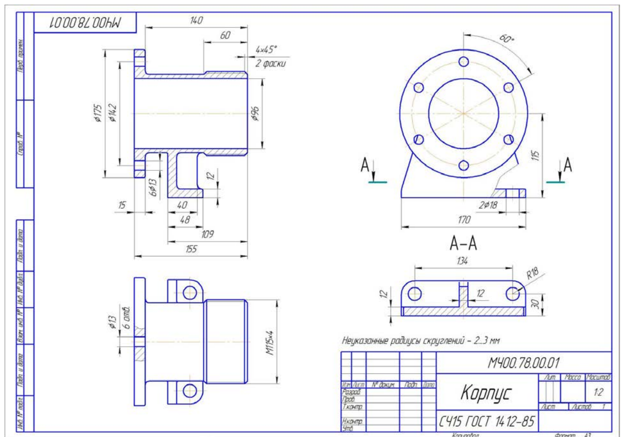
Рис. 8. «Деталирование». Чертежи деталей.
