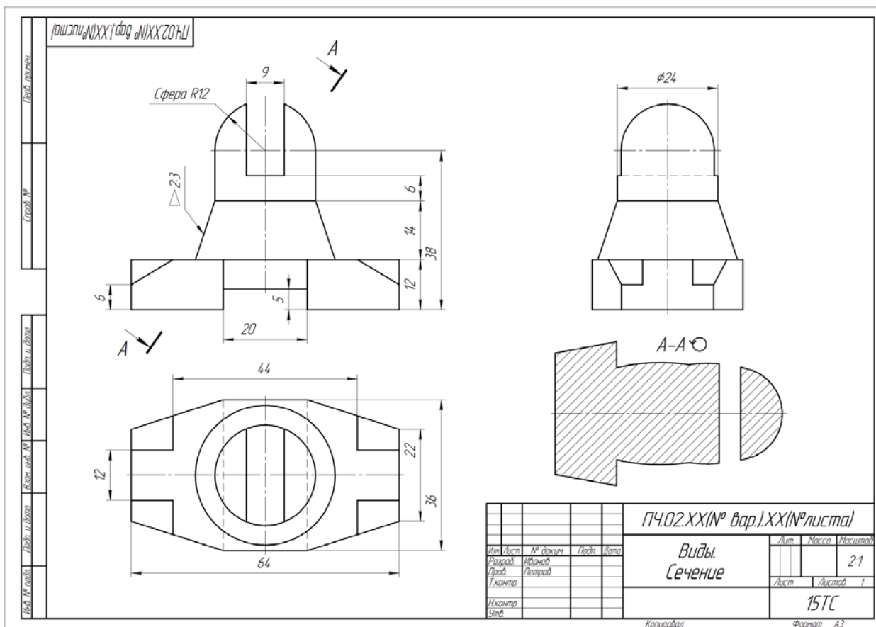
Рис. 3. Построение третьего вида и сечения.
