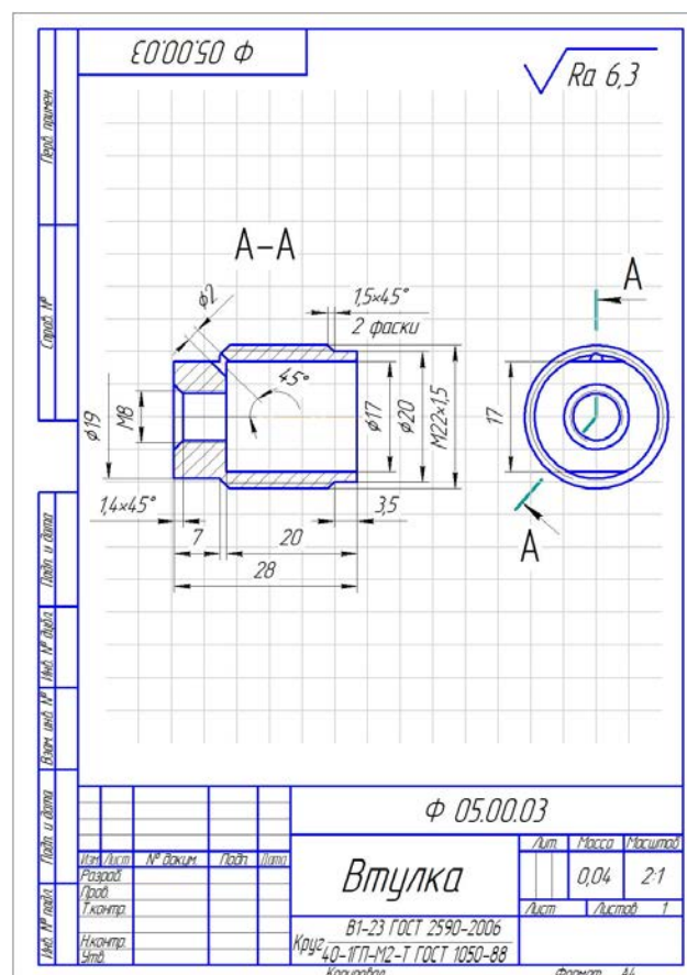
Рис. 7. Спецификация. Эскизы.
