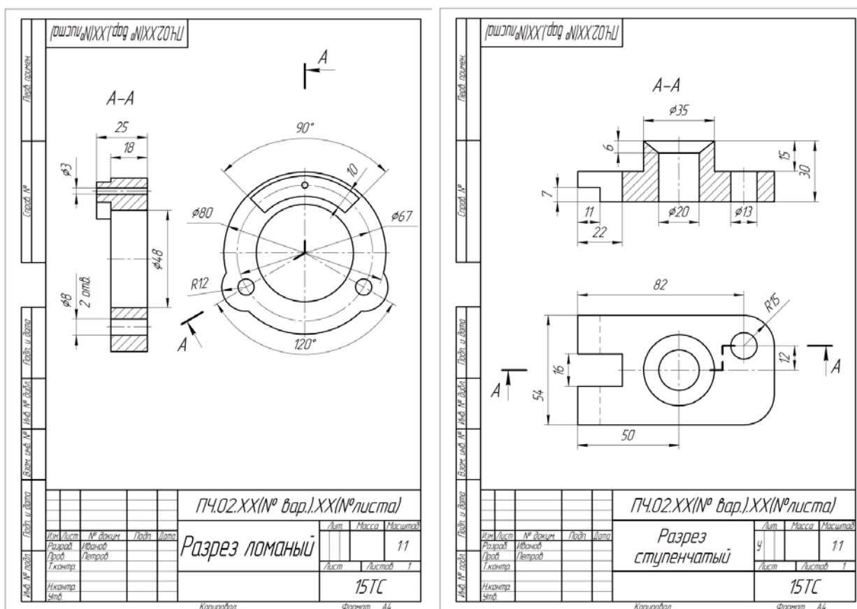
Рис. 5. Сложные разрезы.
