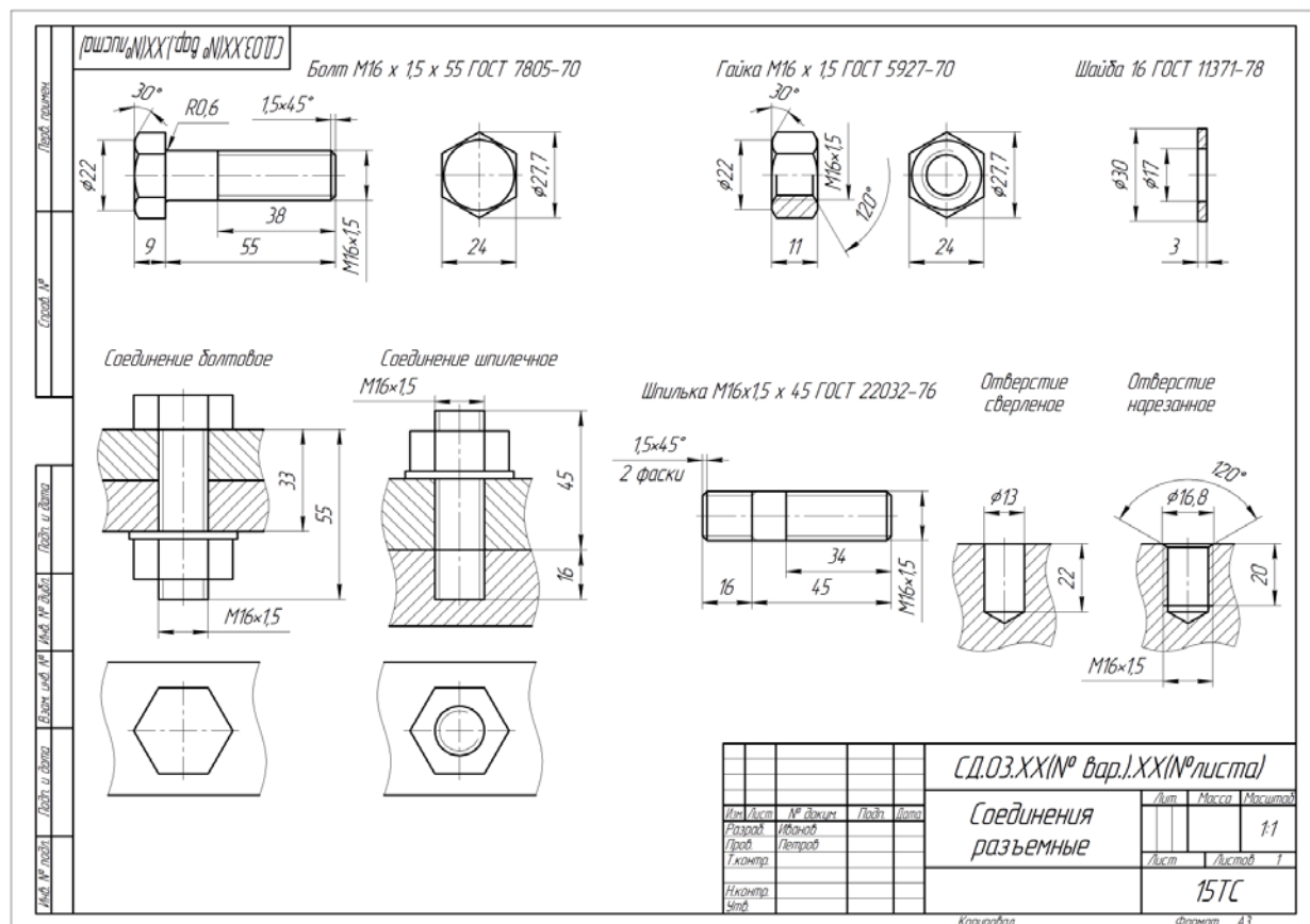
Рис. 6. Соединения разъемные резьбовые.
