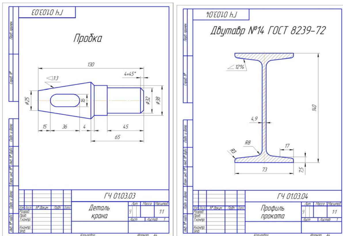
Рис. 2. Конусность. Уклон.
