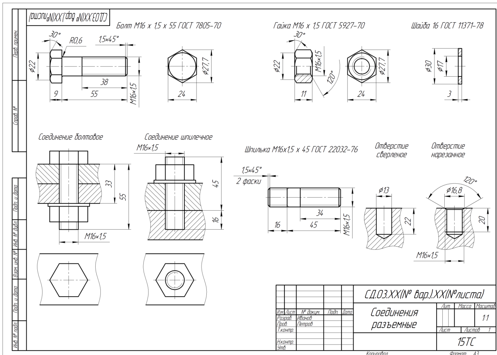
Рис. 8. Графическая работа «Соединения деталей» (Лист 10 – Соединения резьбовые)
