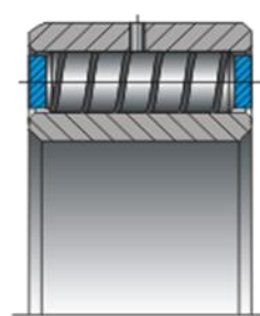
3) роликовый подшипник
